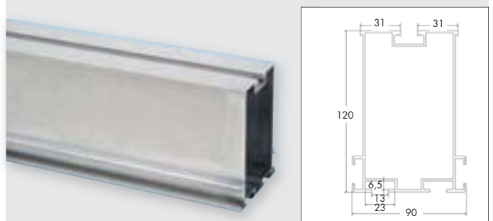
Profilato Solar 120 x 90
