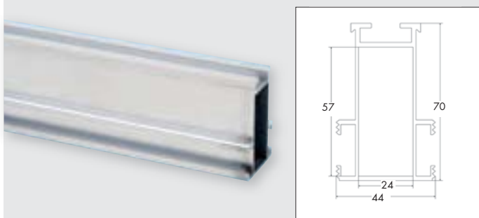
Profilato Solar 70 x 44
